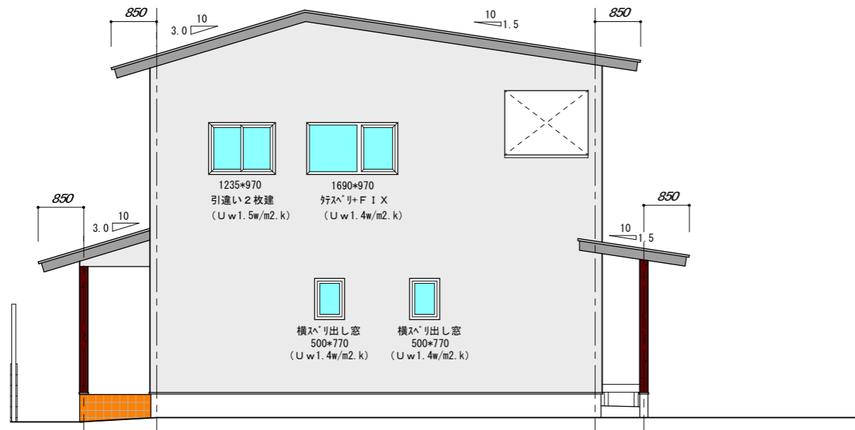
西側立面図
