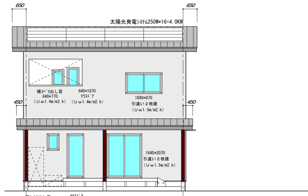
南側立面図
