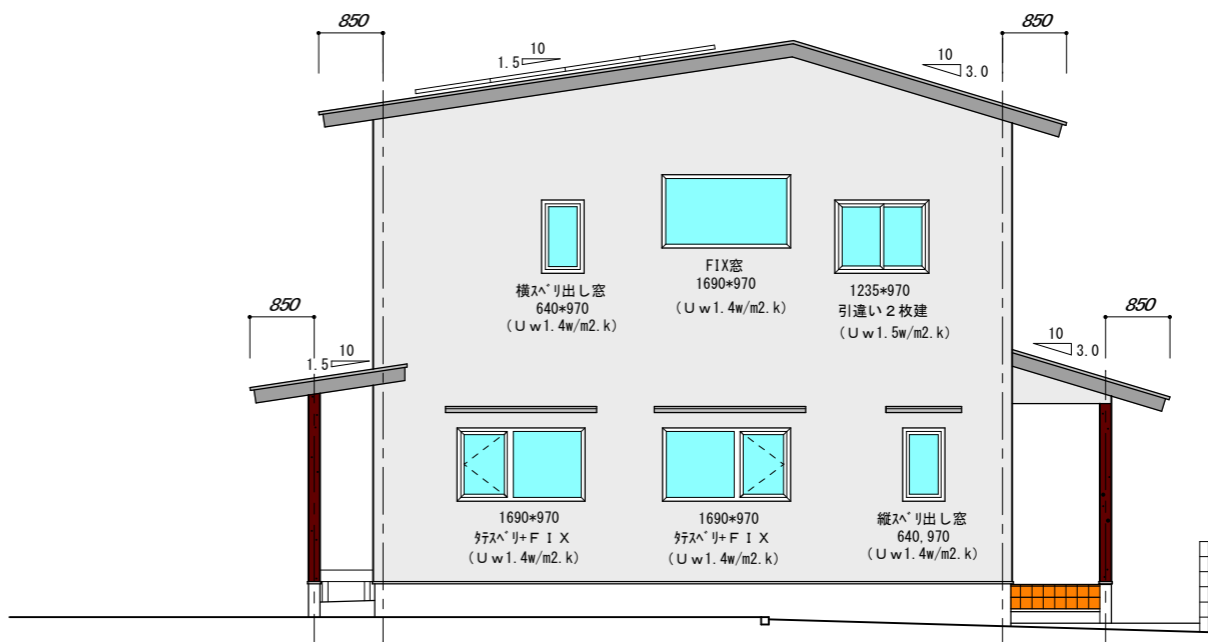
東側立面図
